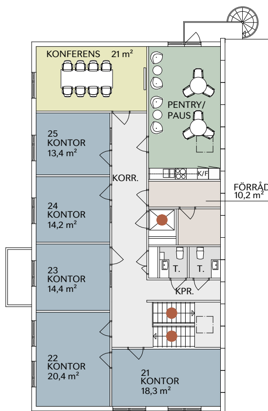
PLAN 2, OVANVÅNING
