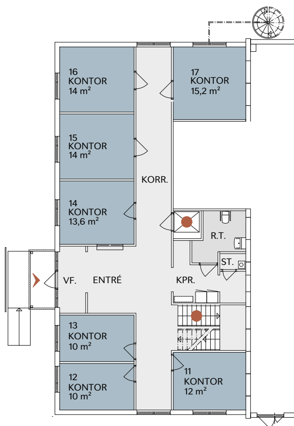
PL AN 1 BOTTENVÅNING
