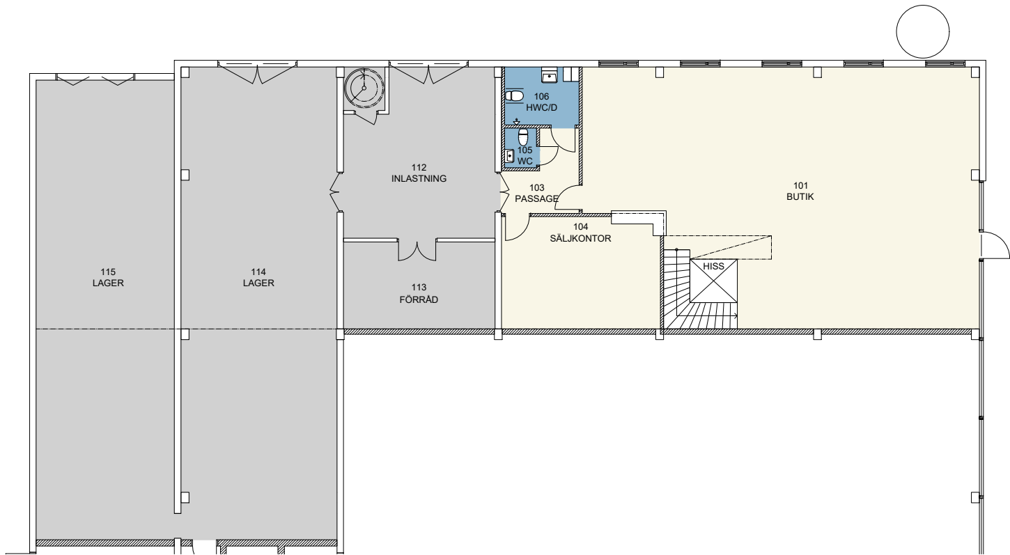
Plan 1, Entréplan
