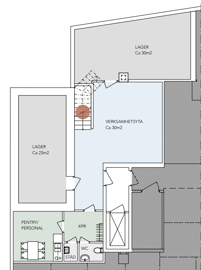
KÄLLARPLAN
