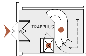
VÅNING 1, ENTRÉPLAN
