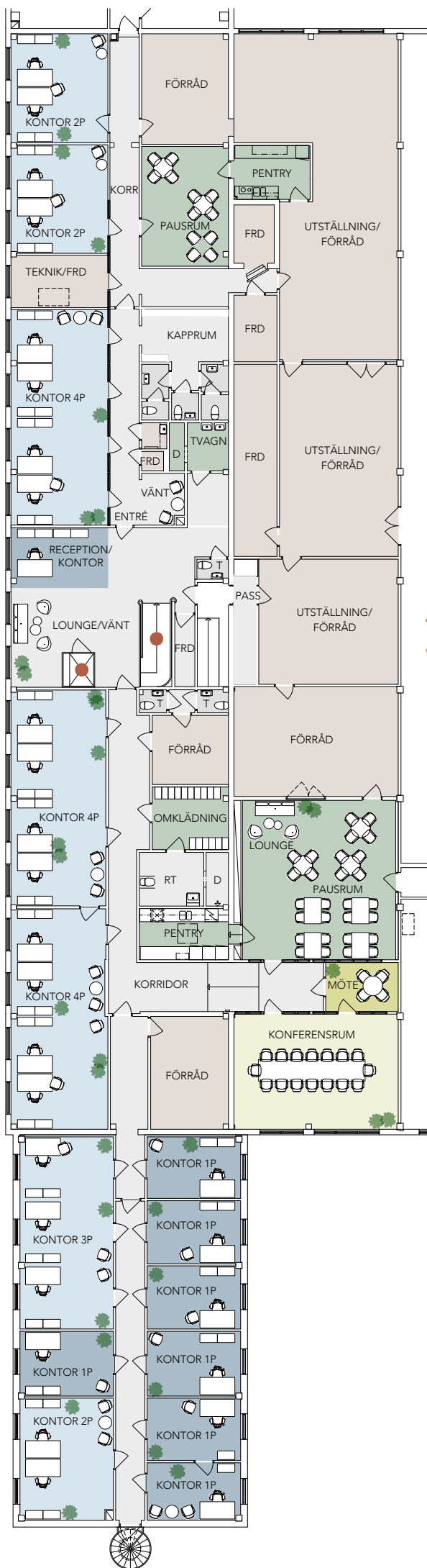
VÅNING 1, ENTRÉPLAN
