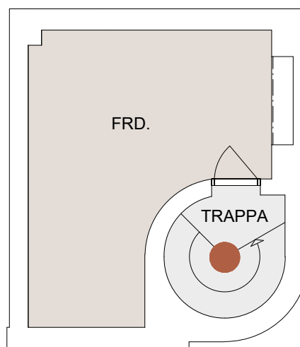
PLAN 0, KÄLLARE
