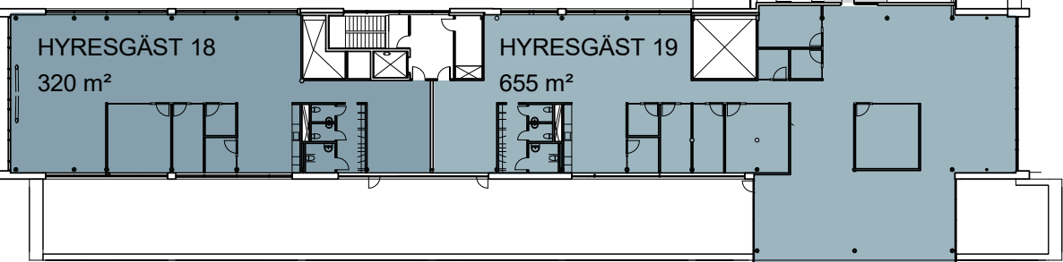
PLAN 14 (vån 5)
