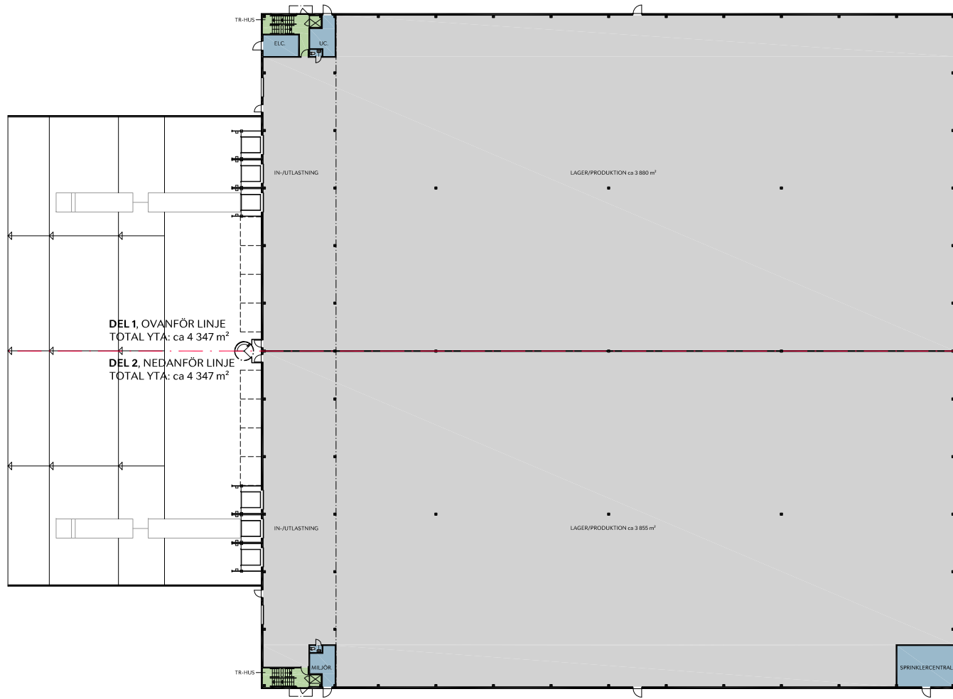
PLAN 10, BOTTENVÅNING
