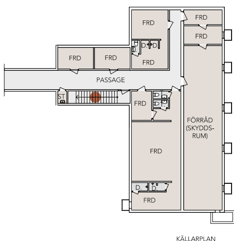
KÄLLARPLAN
