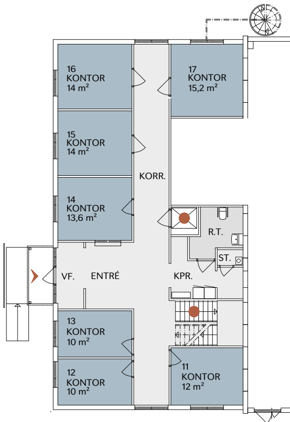
PLAN AN 1 BOTTENVÅNING
